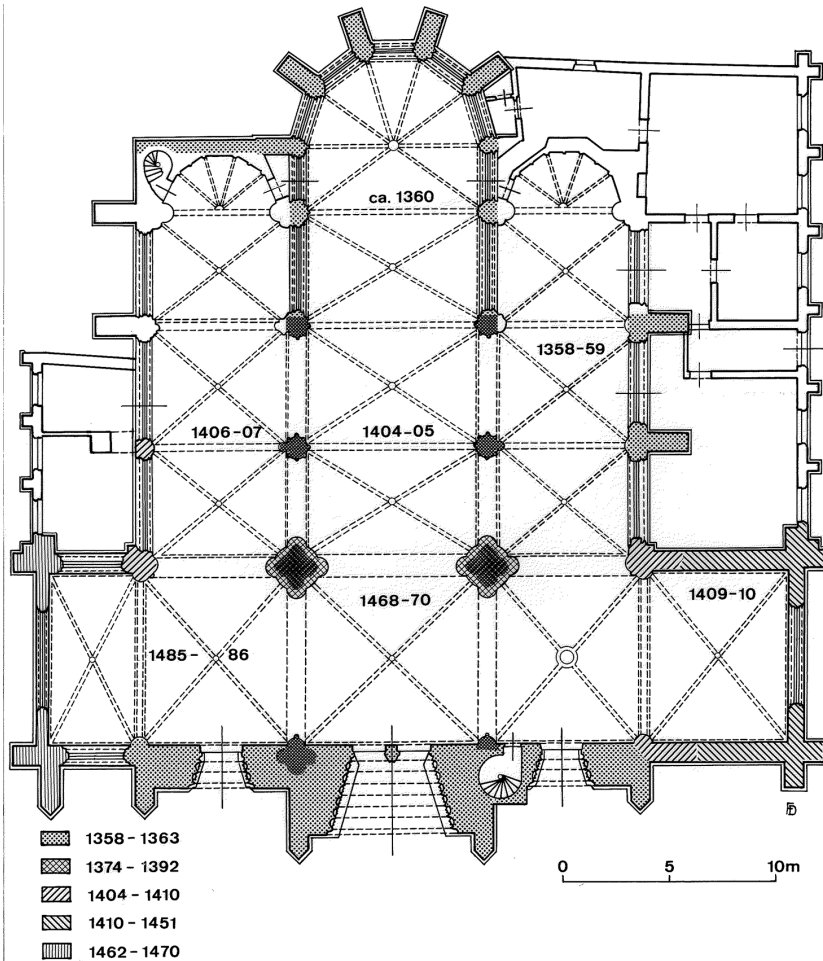
Tienen, Onze-Lieve-Vrouw-ten-Poelkerk, grondplan (tekening : F. Doperé).
